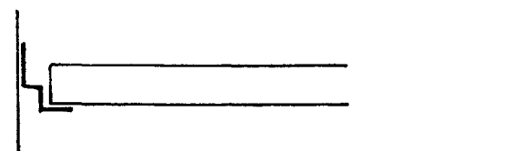
Vegganslutning med skyggefugelist type V-2
