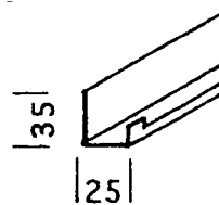
Modullist type V-4 Valgfri modul
