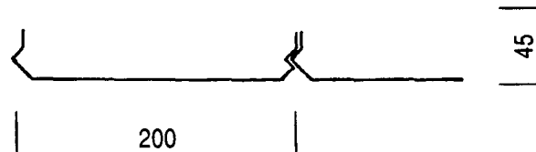
MK-P-T-NP-200
