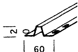
Dobbel hakeskinne 86 med modulerte festenaubber
