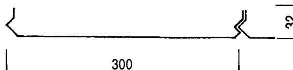
MK-P-T-NP-300, modul 300
