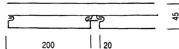
MK-P-T-SP-200
